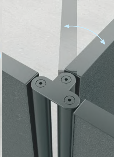
Przegubowe połączenie ścianek Joint connections of walls
