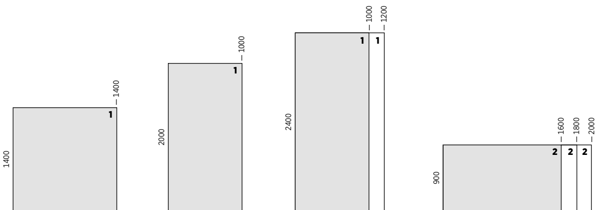
Dimensions of conference tables | Wymiary stołów konferencyjnych
